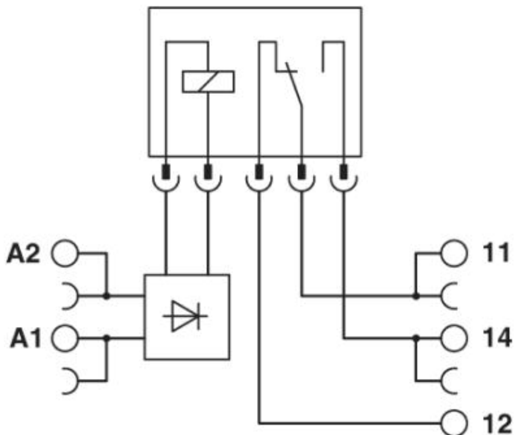
Diagrama eléctrico
