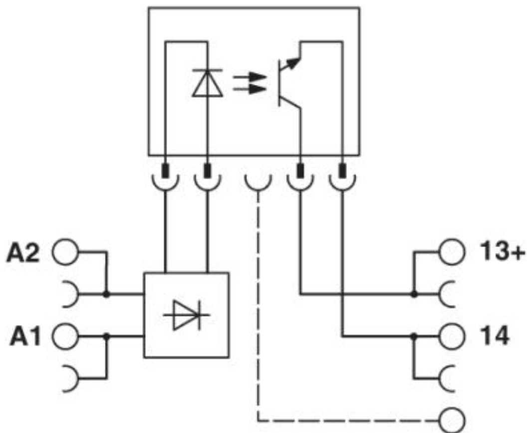
Diagrama eléctrico
