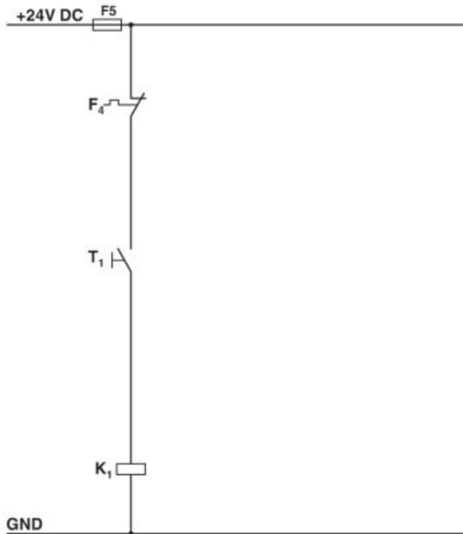
Diagrama eléctrico
