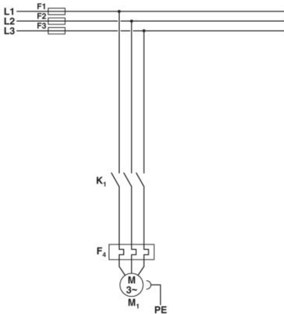
Diagrama eléctrico
