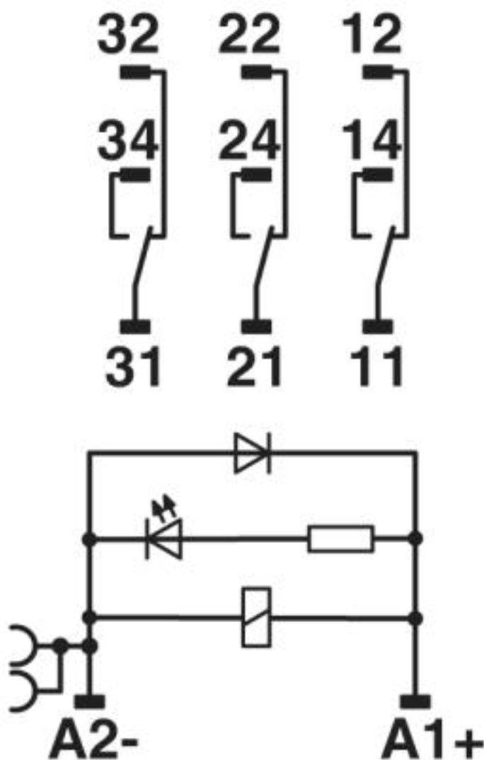
Diagrama eléctrico
