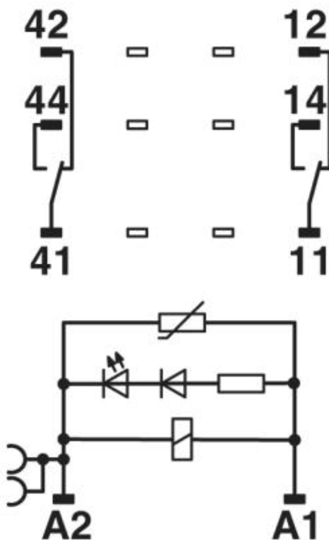
Diagrama eléctrico
