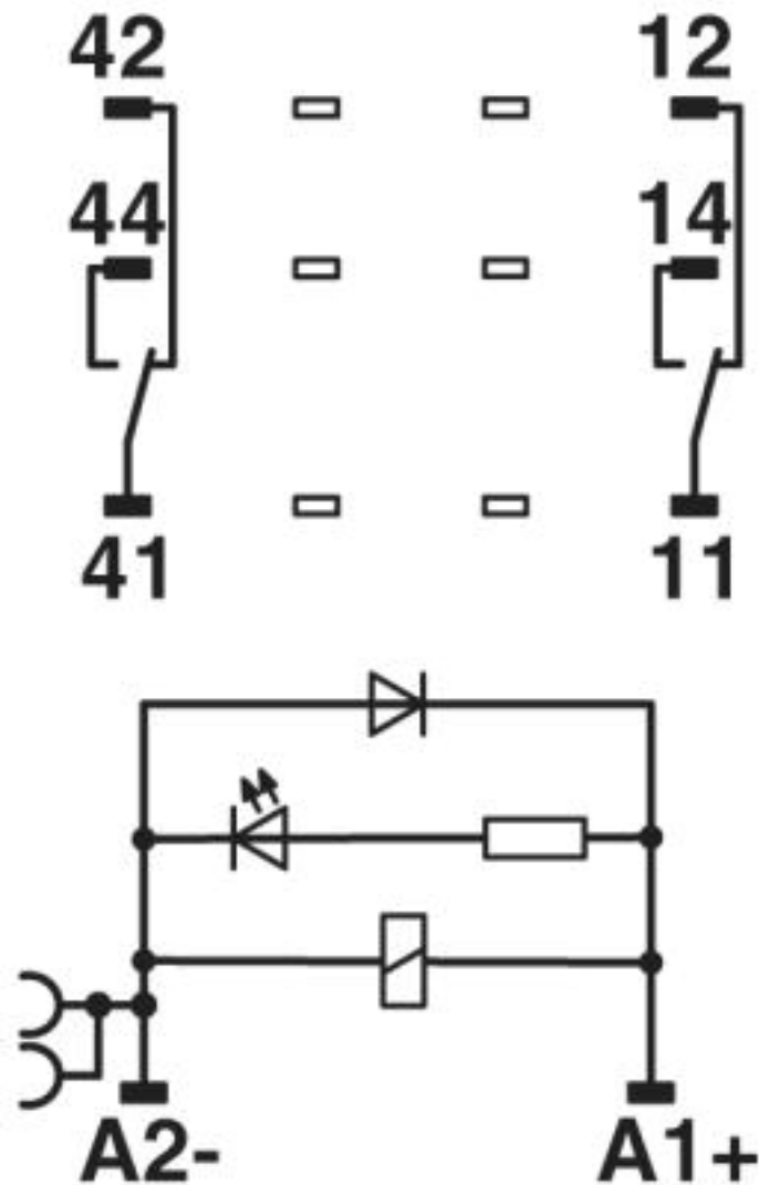
Diagrama eléctrico
