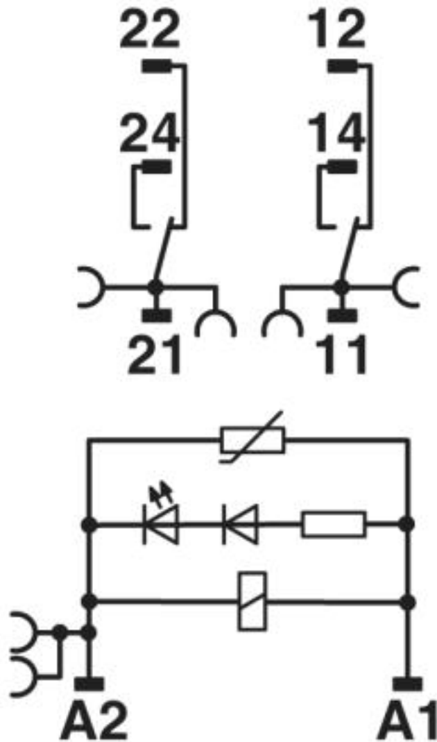
Diagrama eléctrico
