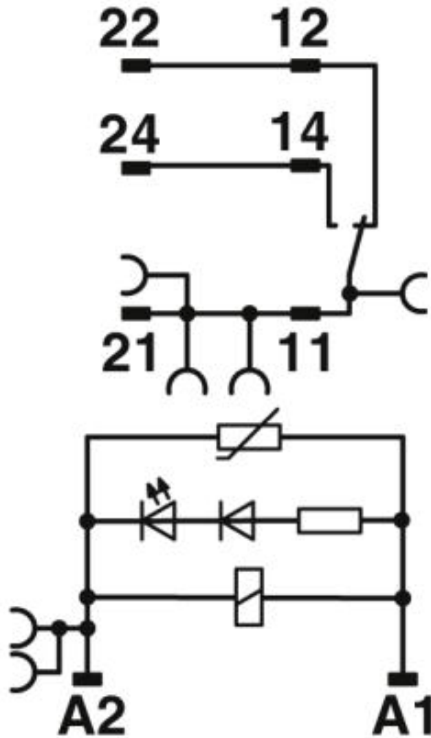
Diagrama eléctrico
