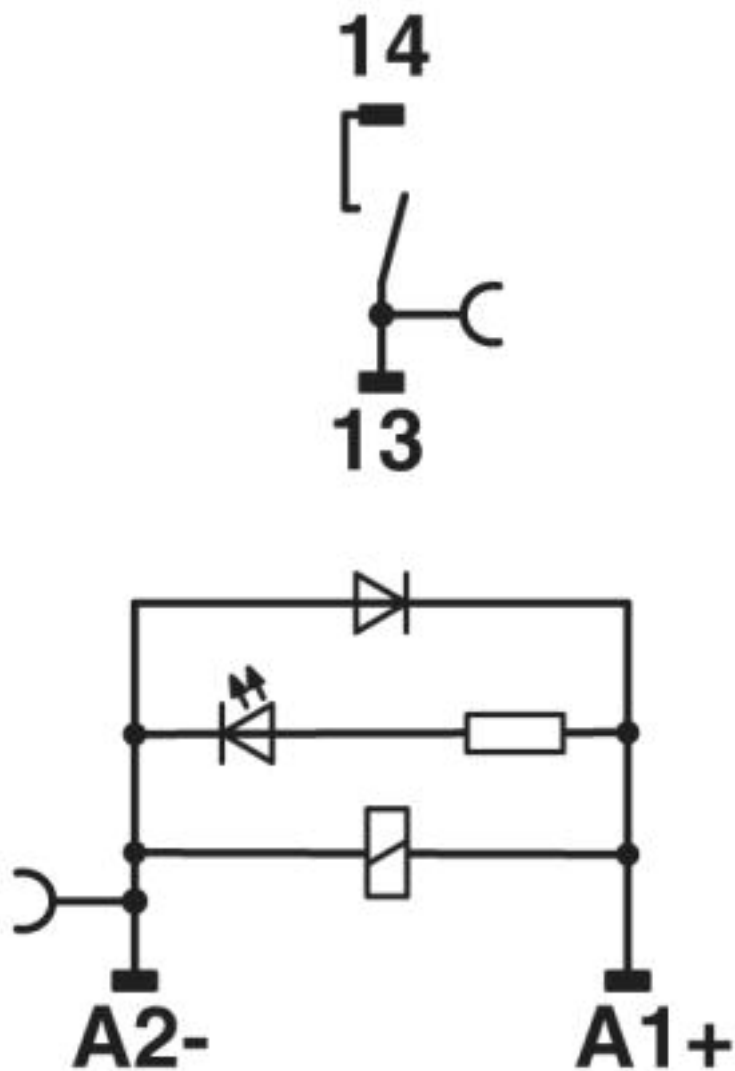
Diagrama eléctrico
