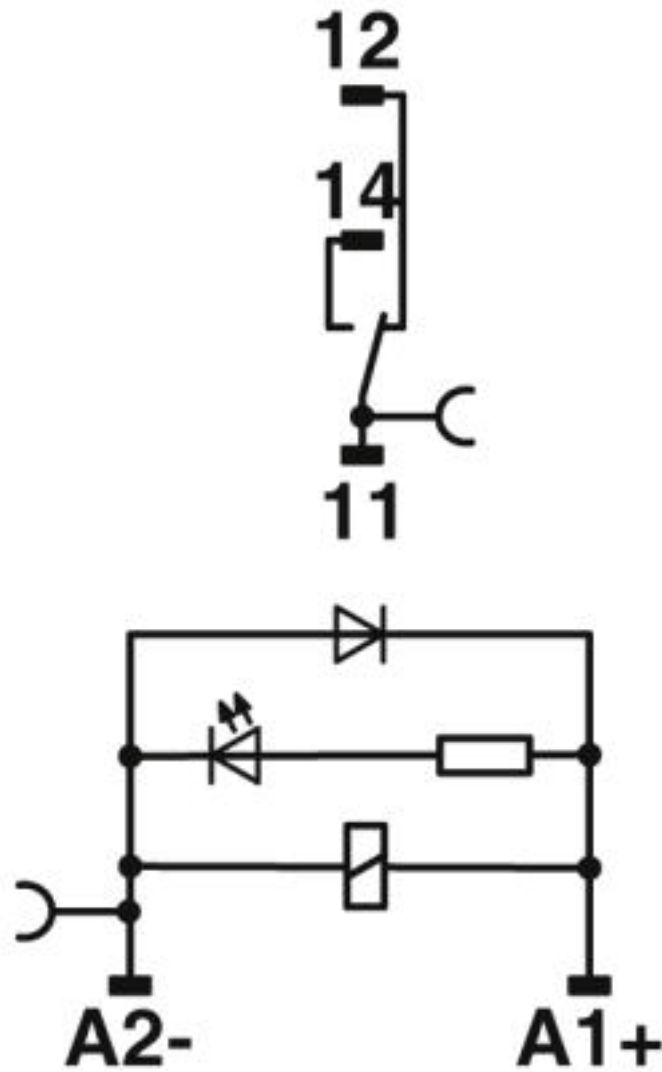
Diagrama eléctrico
