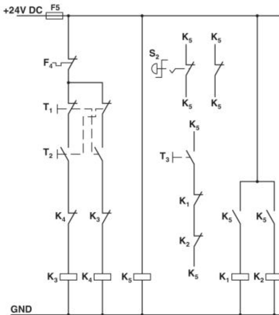
Diagrama eléctrico
