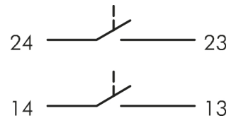
Esquema eléctrico:
