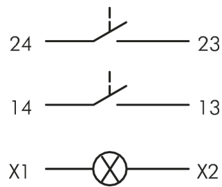
Esquema eléctrico:
