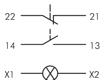
Esquema eléctrico:
