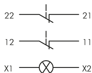
Esquema eléctrico:
