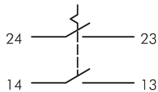
Esquema eléctrico:
