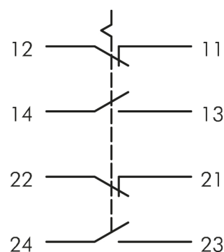
Esquema eléctrico:
