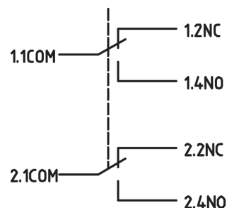
Esquema eléctrico:
