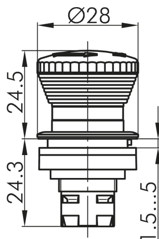
Dimensiones:
