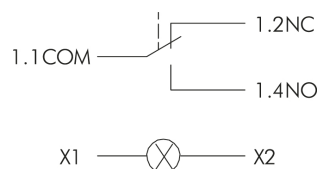
Esquema eléctrico:
