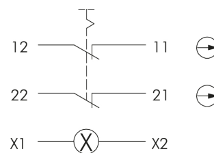
Esquema eléctrico:
