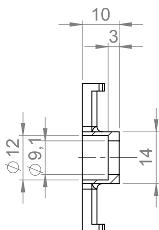
SCHNITT A-A
