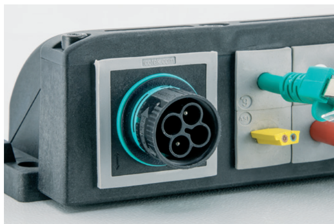
Los marcos permiten el montaje de los insertos adaptadores modulares.
