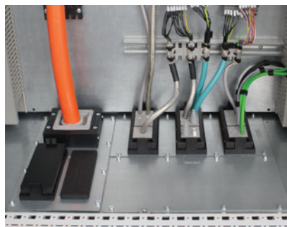
Entrada de cables usando placas modulares en un armario TS 8. Montaje con placa icotek KDR-BMP
